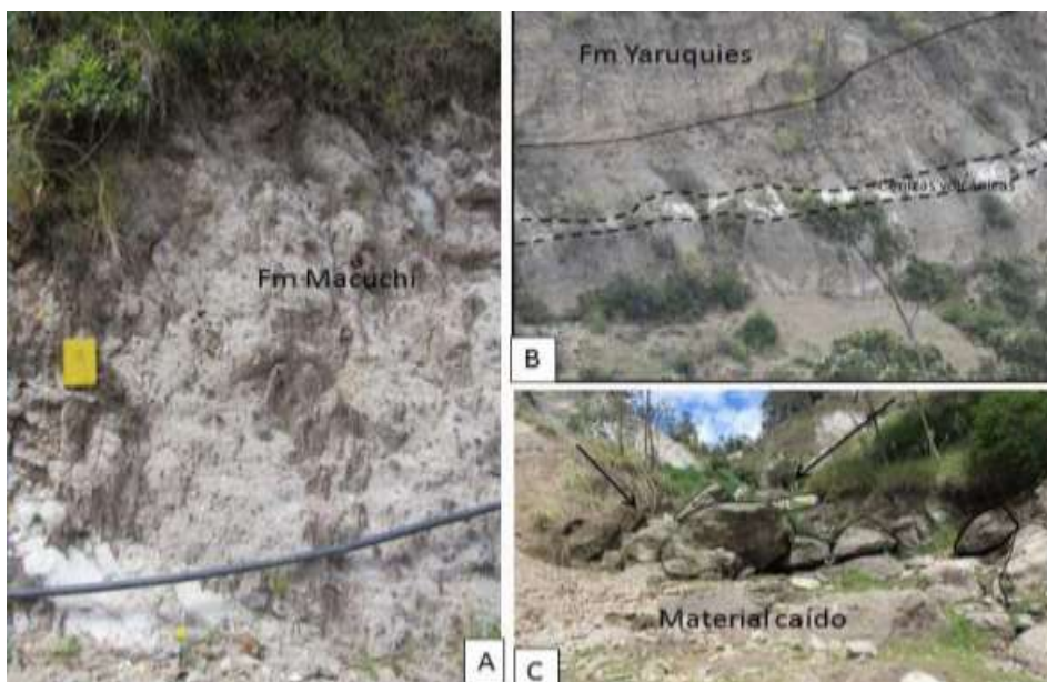
Imagen 1. Formaciones geológicas de la parroquia Cacha
